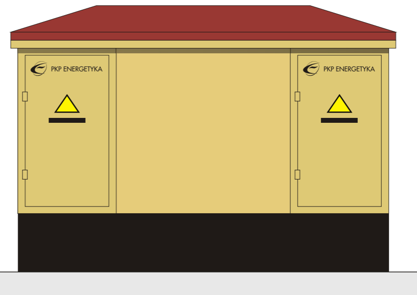
stacja transformatorowa lubelska małogabarytowa w obudowie betonowej typu STLmb-5
